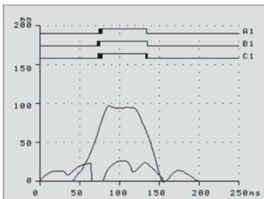
合--分闸测试图形
