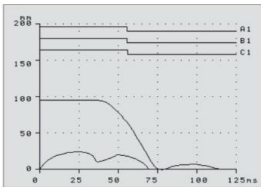
分闸测试图形
