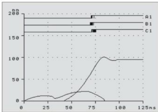
合闸测试图形
